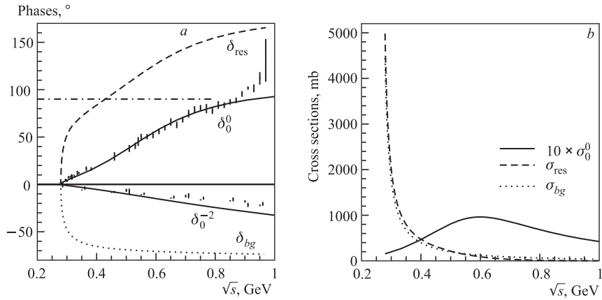
Fig. 2. \delta_0^0 = \delta_{\text{res}} + \delta_{bg}
