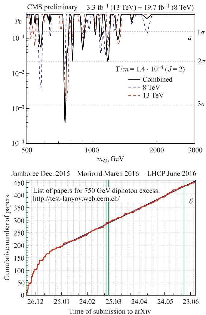
Рис. 4. a ) Вероятность флуктуации фона СМ до наблюдаемого уровня сигнала как функция массы тяжелых дифотонных резонансов отдельно для данных при 8 и 13 ТэВ и их комбинации [4]. б ) Рост полного числа научных работ по превышению в дифотонных спектрах при m = 750 ГэВ в архиве препринтов arXiv в зависимости от времени
