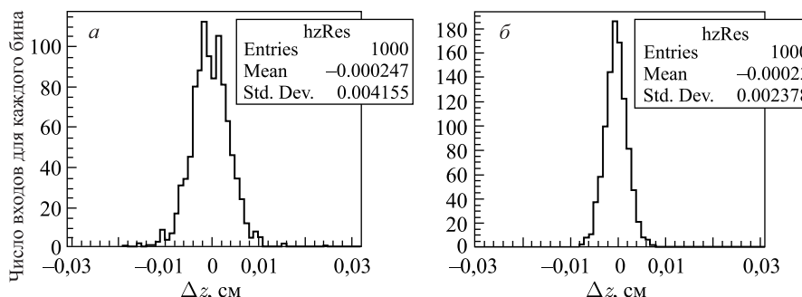
Рис. 4. Зависимость точности реконструкции z -координаты первичной вершины взаимодействия от импульса первичной частицы: а) 1 ГэВ/с; б) 3 ГэВ/с
