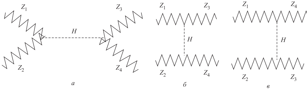
Рис. 7. Диаграммы, описывающие упругое рассеяние Z -бозонов
