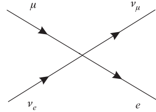
Рис. 1. Распад мюона в локальной 4-фермионной теории
