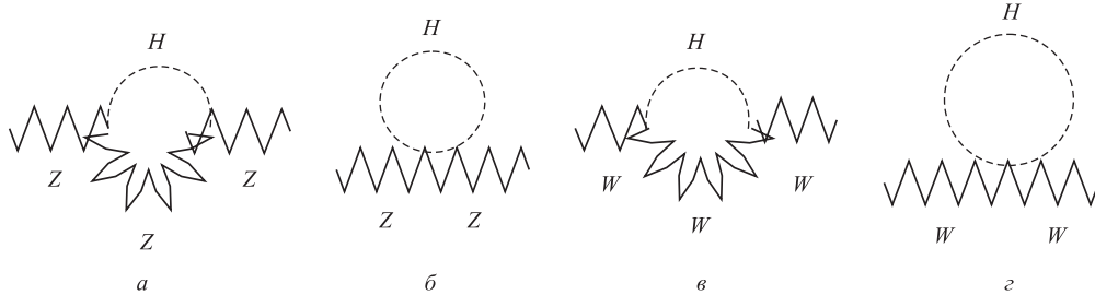
Рис. 16. Вклад хиггсовского бозона в поляризионные операторы векторных бозонов
