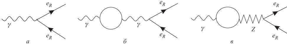
Рис. 11. Графики, перенормирующие затравочный заряд правого электрона
