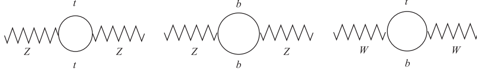
Рис. 15. Графики, приводящие к усиленному как (m_t/m_Z)^2 вкладу в электрослабые радиационные поправки
