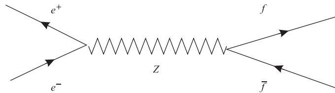
Рис. 6. Рождение Z -бозона с последующим распадом на пару f\bar{f} в e^+e^- -аннигиляции (ускорители SLC и LEP I)
