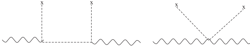
Рис. 4. Две диаграммы, описывающие вклад \sim e^2 в поляризационный оператор векторного бозона
