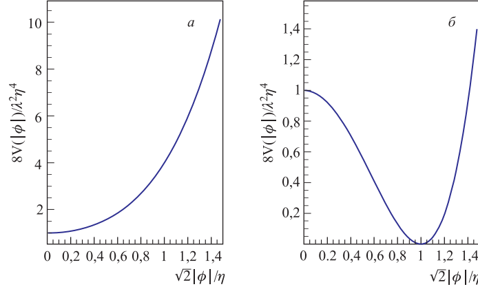
Рис. 3. Обычная (а) и приводящая к эффекту Голдстоуна (б) зависимости плотности потенциальной энергии от безразмерной величины \sqrt{2}|\phi|/\eta
