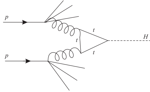
Рис. 8. Рождение хиггса в pp -столкновениях
