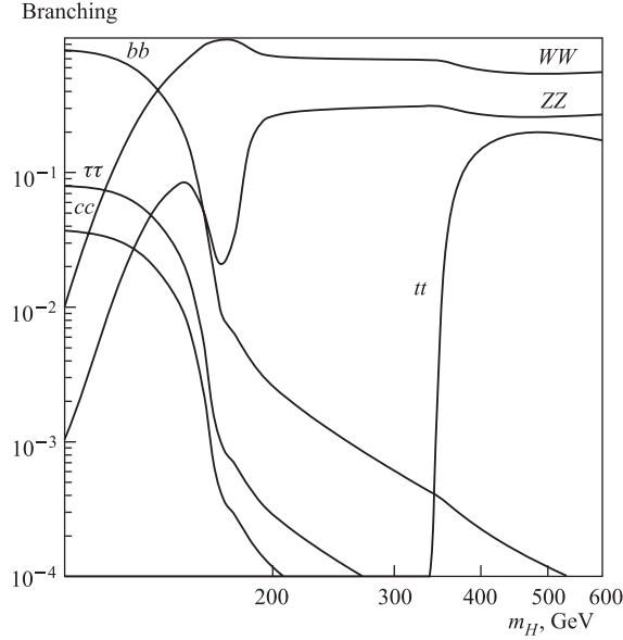
Рис. 10. Относительные вероятности распадов H
