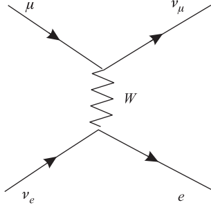
Рис. 2. Распад мюона в теории с промежуточным векторным бозоном
