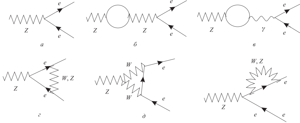
Рис. 13. Амплитуда распада Z \rightarrow e^+e^- с учетом петлевых поправок
