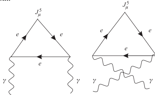
Рис. 5. Диаграммы, приводящие к несохранению аксиального тока в квантовой электродинамике с безмассовым электроном
