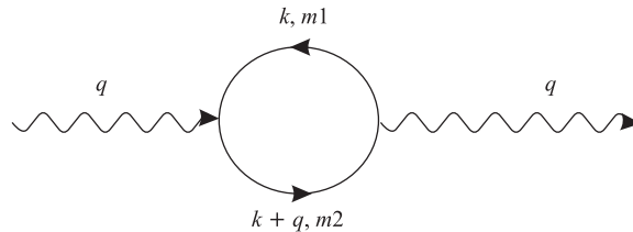
Рис. 14. Вклад фермионной петли в поляризационный оператор векторных бозонов
