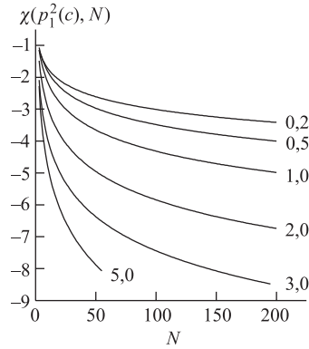
Рис. 2. Десятичный логарифм (39) относительной точности аппроксимации p_1^2(c) \approx \tilde{p}_1^2(c) собственного значения p_1^2(c) как функция верхнего индекса N суммы (38) при значениях параметра c , указанных цифрами у кривых
