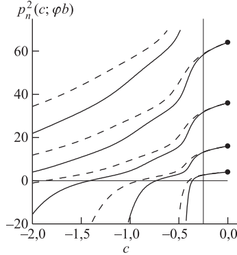
Рис. 3. Собственные значения в «обрезанном» в точке \varphi_b = \pi/2 - s_b поле (1): сплошные кривые — при s_b = (\pi/2)/999 , штрихпунктирные — при s_b = (\pi/2)/300 ; тонкие сплошные горизонтальная и вертикальная линии — прямые p^2 = 0 и c = -1/4 ; символом \bullet обозначена точка с координатами c = 0 и p_n^2 = (2n)^2 , n = 1, 2, 3, 4
