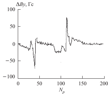
Рис. 7. График разности \Delta B_y величин \overline{B}(x, y, z) и B_y(x, y, z + \Delta z) для осевой линии ( x=y=0 )
