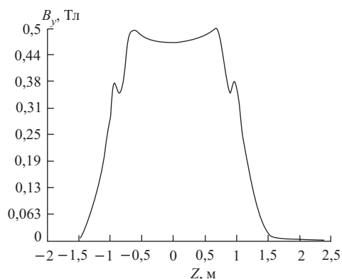
Рис. 13. График B_y = B_y(x = -0,55 \text{ м}; y = -0,3 \text{ м}; z) в зависимости от продольной координаты z
