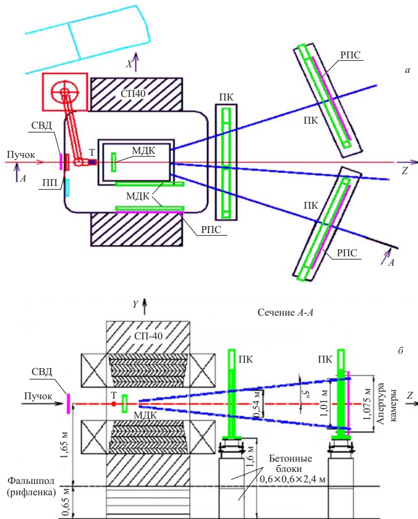
Рис. 1. Схема установки НИС: а) горизонтальная ZOX -плоскость. Т — жидководородная мишень; ПК — пропорциональная камера; МДК — мини-дрейфовая камера; РПС — резистивные плоские счетчики; СВД — сцинтилляционный волоконный датчик; ПП — профилометр пучка; СП-40 — анализирующий магнит; б) вертикальный разрез, ZOY -плоскость
