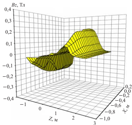
Рис. 12. Поверхность B_z = B_z(x, y = -0,3 \text{ м}; z) для плоскости P1 , y=-0,3 \text{ м}
