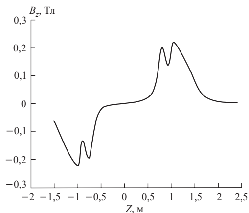
Рис. 15. График B_z = B_z(x = -0,55 м; y = -0,3 м; z) в зависимости от продольной координаты z
