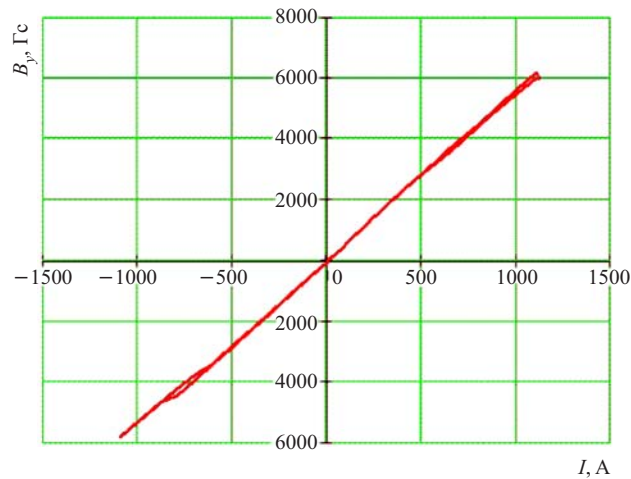
Рис. 5. Кривая возбуждения B = B(I) для магнита 1СП-40-4В
