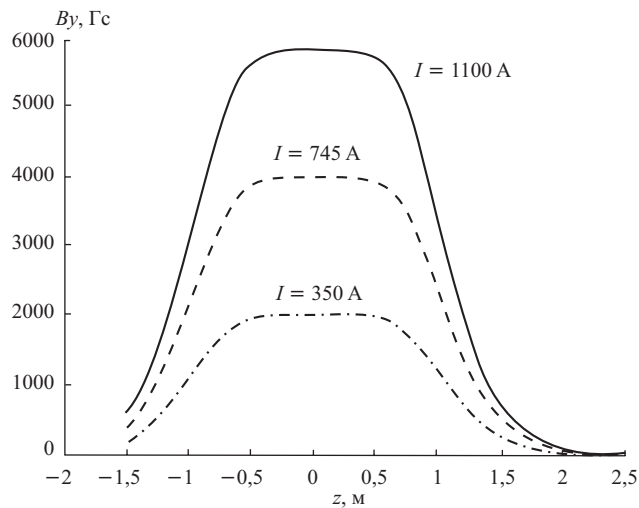
Рис. 8. Зависимость основной компоненты магнитной индукции B_y(0, 0, z) от продольной координаты z при фиксированных x и y для трех значений тока в обмотке магнита
