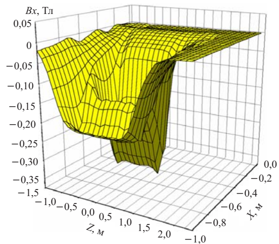
Рис. 11. Поверхность B_x = B_x(x, y = -0,3 \text{ м}; z) для плоскости P1 , y=-0,3 \text{ м}
