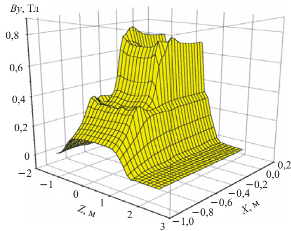
Рис. 10. Поверхность B_y = B_y(x, y = -0,3; z) для плоскости P1, y=-0,3 \text{ м}
