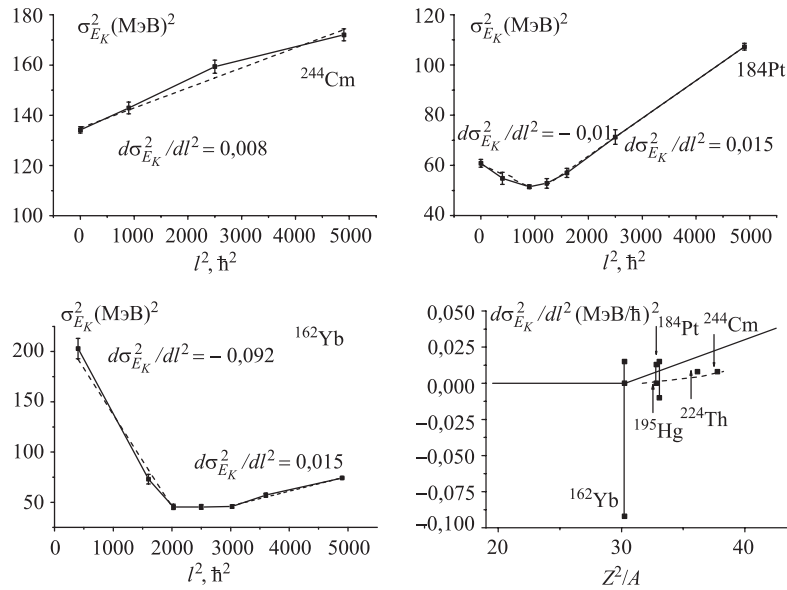
Рис. 4. Зависимость дисперсии энергетического распределения от l^2 для ^{244}\text{Cm} , ^{184}\text{Pt} и ^{162}\text{Yb} (сплошная линия) и линейная аппроксимация зависимости (штриховая линия). Рядом указаны коэффициенты линейной аппроксимации. Остальные обозначения — аналогично рис. 3
