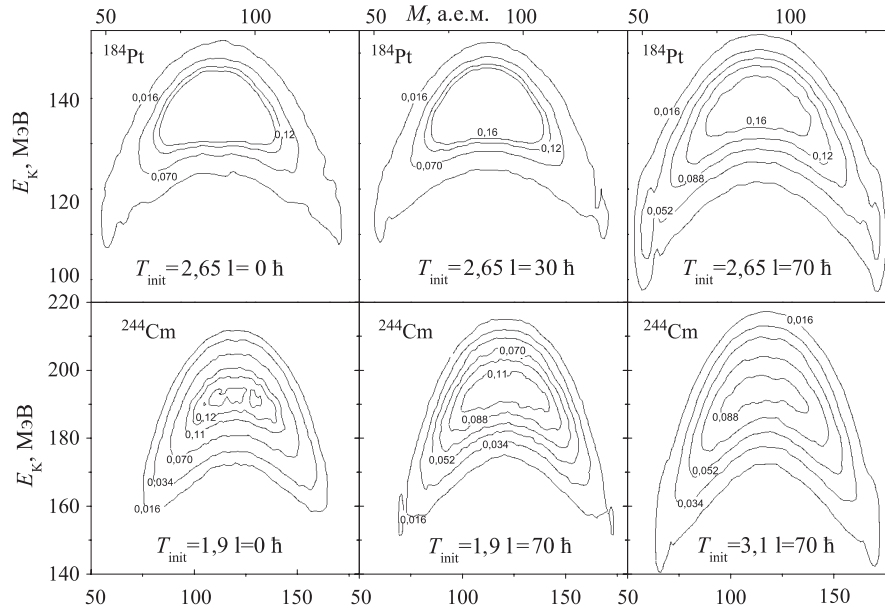
Рис. 1. Двумерные карты массово-энергетических распределений для ^{184}\text{Pt} при T_{\text{init}} = 2,65 МэВ и разных значениях величины углового момента, а также ядра ^{244}\text{Cm} при T_{\text{init}} = 1,9 и 3,1 МэВ и двух значениях l = 0 и 70 \hbar . Цифры при линиях — выход осколков в процентах. Полный выход нормирован на 200 %
