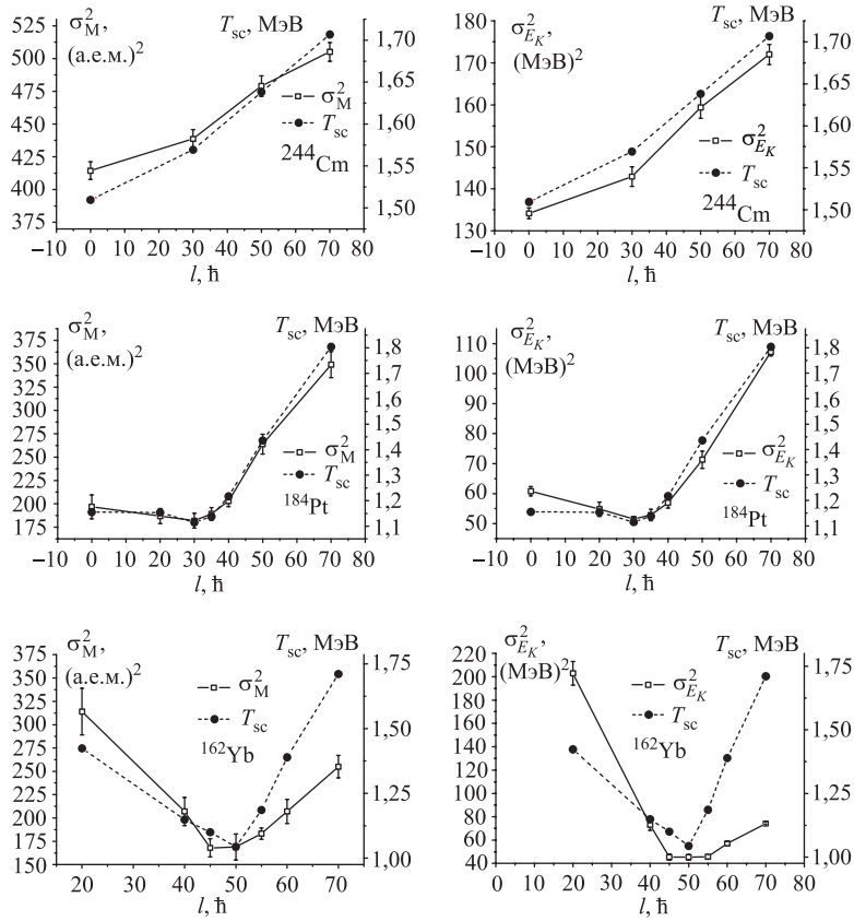
Рис. 5. Дисперсии массового (слева) и энергетического (справа) распределений (открытые квадраты) и температура в разрыве (круги) для ^{244}\text{Cm} , ^{184}\text{Pt} , and ^{162}\text{Yb} как функция углового момента
