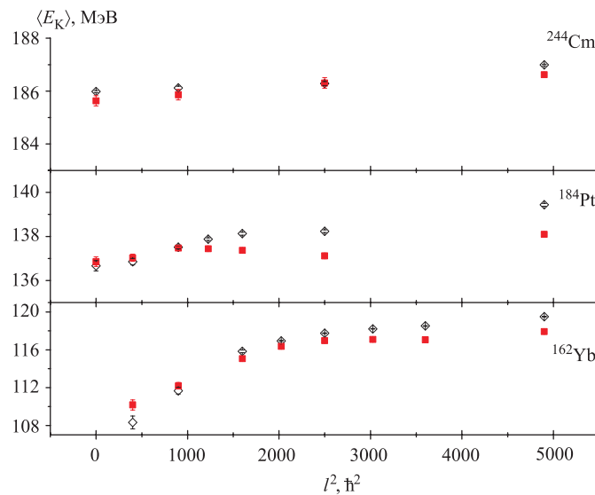
Рис. 2. Средняя кинетическая энергия для трех составных систем Cm, Pt и Yb при двух значениях исходных температур как функция углового момента. Открытыми ромбами показаны значения \langle E_K \rangle при T = 2 \text{ МэВ} , закрашенными квадратами — при T = 3,1 \text{ МэВ}
