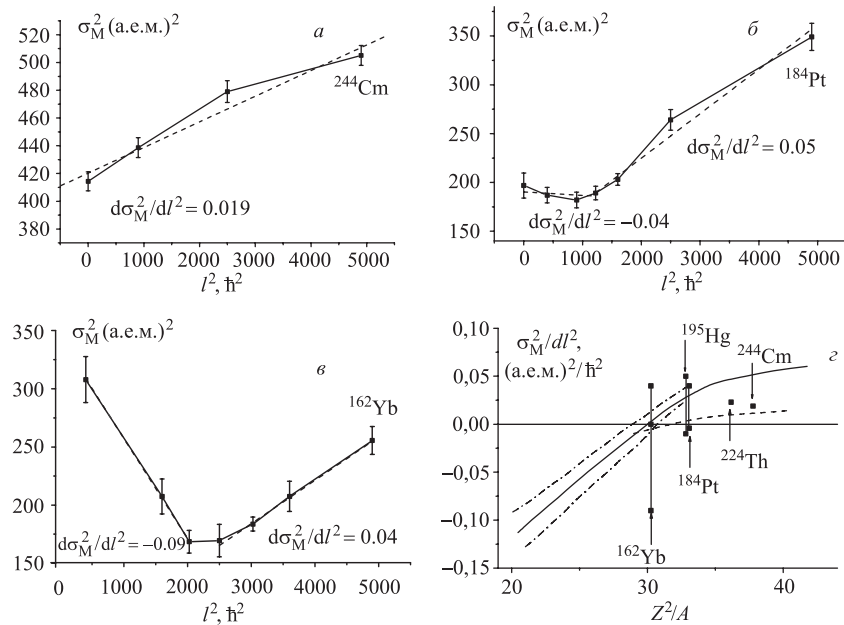
Рис. 3. а–в) Зависимость дисперсии массового распределения от l^2 для ^{244}\text{Cm} , ^{184}\text{Pt} и ^{162}\text{Yb} (сплошная линия) и линейная аппроксимация зависимости (штриховая линия). Рядом указаны коэффициенты линейной аппроксимации. г) На графике отмечены итоговые результаты в виде зависимости d\sigma_M^2/dl^2 от Z^2/A . Закрашенные квадраты, соединенные линиями, — это результаты наших расчетов. Стрелками указано, какому составному ядру соответствуют данные квадраты. Для каждого из ядер ^{162}\text{Yb} , ^{195}\text{Hg} и ^{184}\text{Pt} несколько покрашенных квадратов соответствуют нескольким значениям коэффициента d\sigma_M^2/dl^2 . Три значения данного коэффициента для ядра ^{162}\text{Yb} и два для ^{184}\text{Pt} отражают изменения в характере зависимости \sigma_M^2 от l^2 . Сплошная кривая — оценка коэффициента d\sigma_M^2/dl^2 на основе экспериментальных данных [7]. Штрихпунктирные кривые показывают пределы погрешности этой оценки. Штриховая кривая — результаты теоретических расчетов группы Адеева с помощью уравнений Фоккера–Планка [12]
