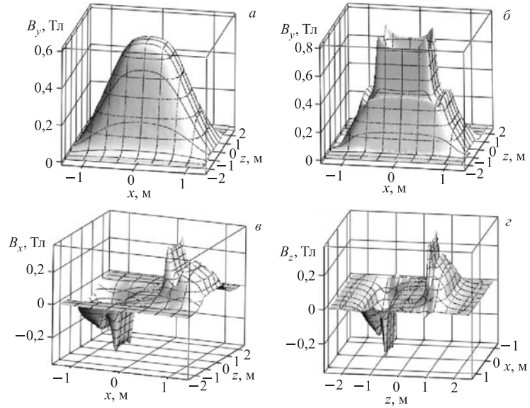
Рис. 3. Зависимости а ) B_y(x, 0, z) ; б ) B_y(x, -0,3 \text{ м}, z) ; в ) B_x(x, -0,3 \text{ м}, z) ; з ) B_z(x, -0,3 \text{ м}, z) для тока 1100 А
