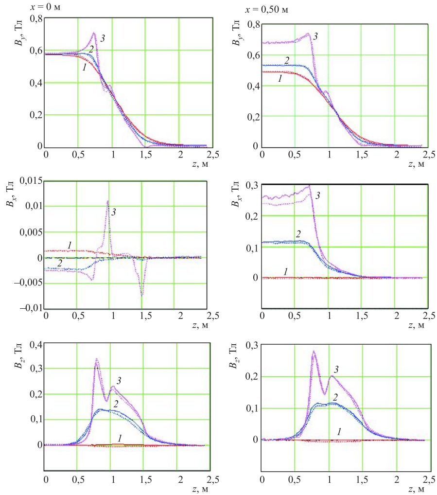
Рис. 7. Зависимости B_y(z) , B_x(z) , B_z(z) для x = 0 (слева) и для x = 0,50 м (справа) для тока 1100 А (сплошные линии — расчет, штриховые — эксперимент; 1 соответствует плоскости y = 0 м, 2 — плоскости y = -0,2 м, 3 — плоскости y = -0,3 м)
