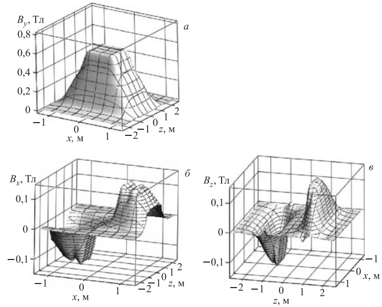
Рис. 4. Зависимости а ) B_y(x, -0,2 \text{ м}, z) ; б ) B_x(x, -0,2 \text{ м}, z) ; в ) B_z(x, -0,2 \text{ м}, z) для тока 1100 А
