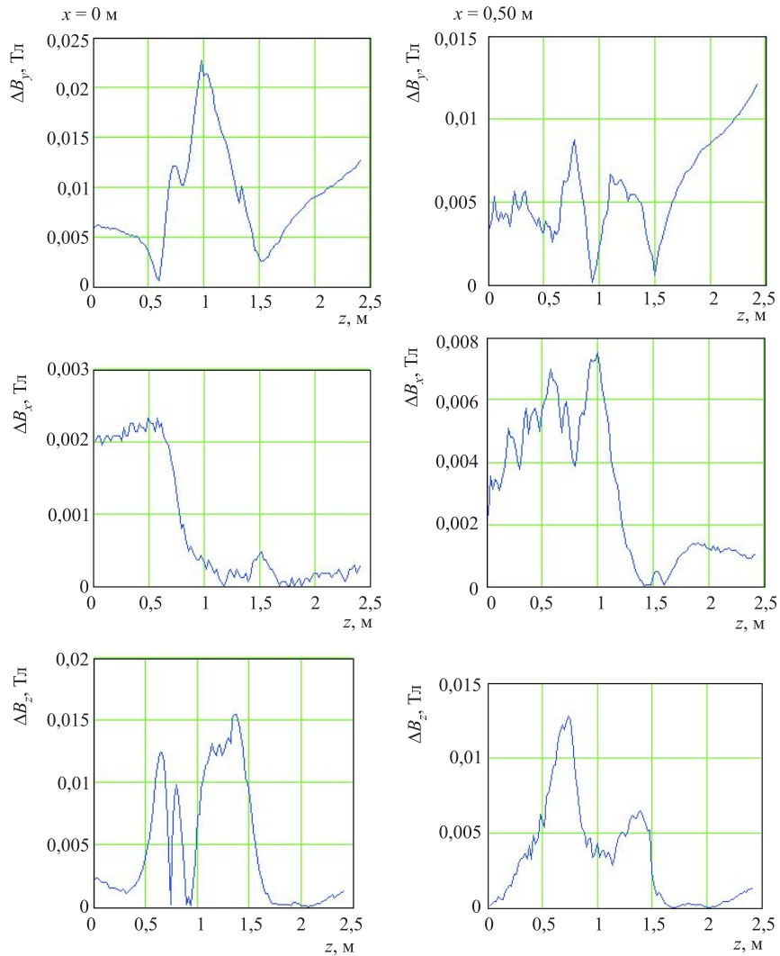
Рис. 9. Разница между экспериментальными и расчетными данными компонент поля для x = 0 (слева) и для x = 0,50 \text{ м} (справа) для тока 1100 А
