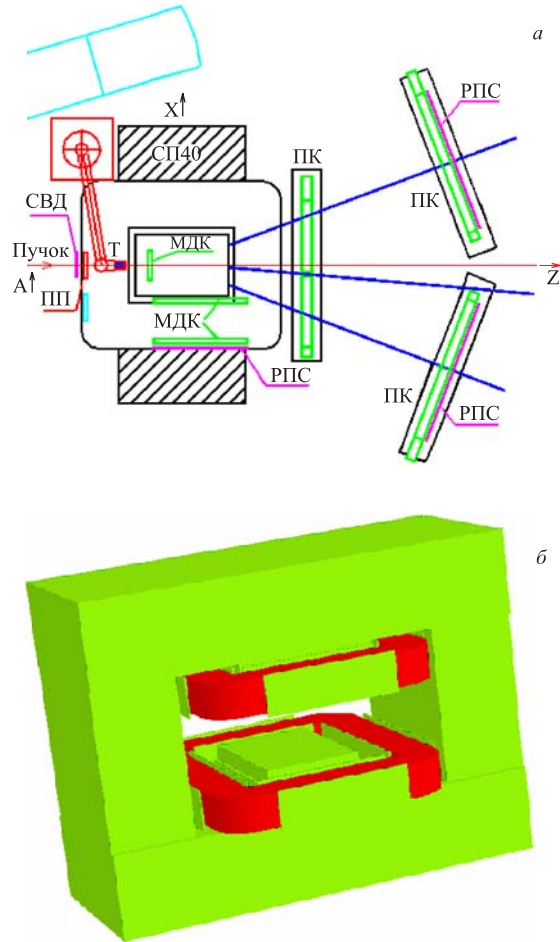
Рис. 1. а ) Схема установки НИС, горизонтальная ZOX-плоскость: Т — жидководородная мишень; ПК — пропорциональная камера; ПП — профилометр пучка; МДК — мини-дрейфовая камера; РПС — резистивные плоские счетчики; СВД — сцинтилляционный волоконный датчик; СП-40 — анализирующий магнит. б ) Общий вид спектрометрического магнита СП-40
