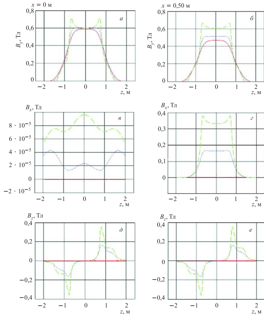
Рис. 5. Зависимости B_y(z) , B_x(z) , B_z(z) для x = 0 (слева) и для x = 0,50 м (справа) для тока 1100 А
