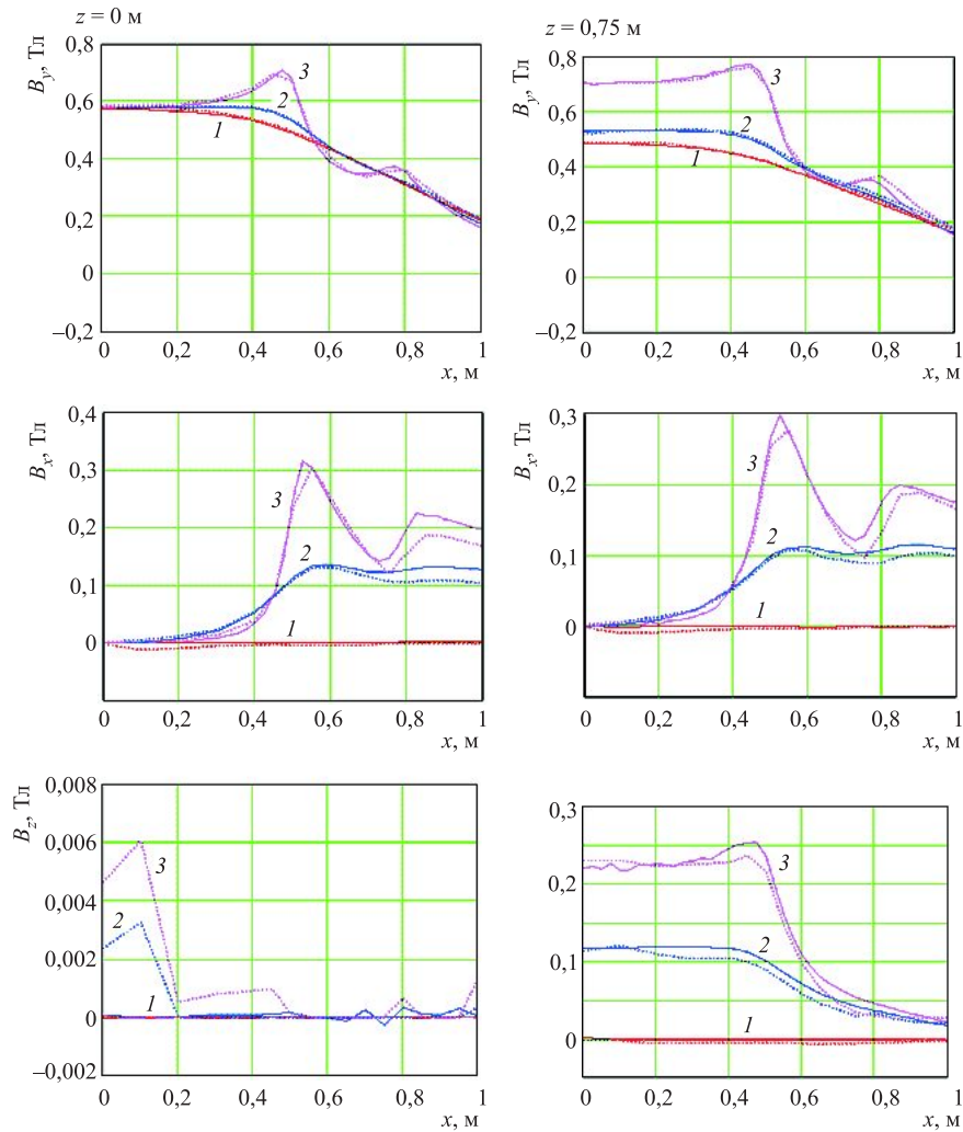
Рис. 8. Зависимости B_y(x) , B_x(x) , B_z(x) для z = 0 (слева) и для z = 0,75 м (справа) для тока 1100 А (сплошные линии — расчет, штриховые — эксперимент; 1 соответствует плоскости y = 0 м, 2 — плоскости y = -0,2 м, 3 — плоскости y = -0,3 м)
