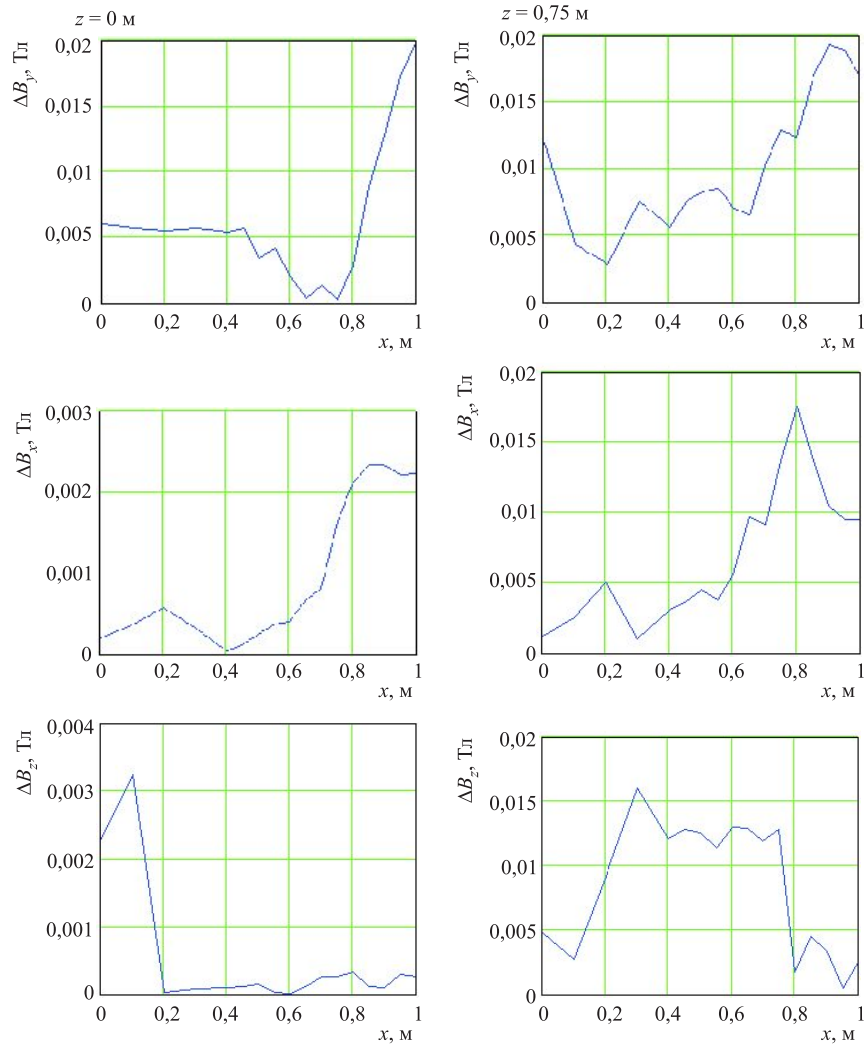
Рис. 10. Разница между экспериментальными и расчетными данными компонент поля для z = 0 (слева) и для z = 0,75 м (справа) для тока 1100 А
