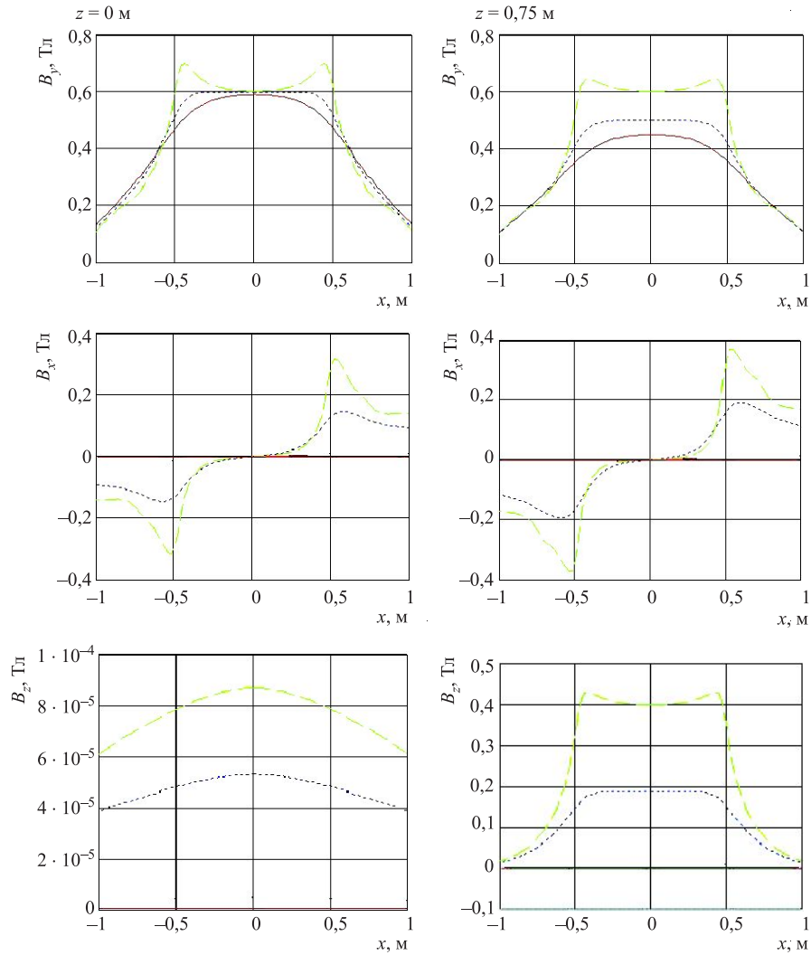
Рис. 6. Зависимости B_y(x) , B_x(x) , B_z(x) для z = 0 (слева) и для z = 0.75 м (справа) для тока 1100 А (сплошная линия соответствует плоскости y = 0 м, штриховая линия — y = -0,2 м, пунктирная линия — y = -0,3 м)
