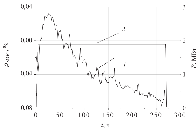
Рис. 1. Реактивность мощностной обратной связи в июльском цикле 1995 г. (1 — реактивность, 2 — мощность)
