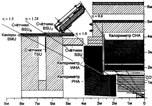
Рис. 17. Расположение детекторов мюонного триггера в области 1.0 \leq |\eta| \leq 1.5 , а также место предполагаемой установки нового слоя сцинтилляционных счётчиков SSU.
