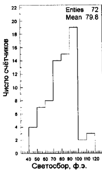
Рис. 10. Светосбор с центра синцилляционной пластины для счётчиков MSK.
