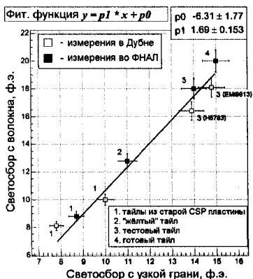
Рис. 14. Корреляция светосбора со спектросмещающего оптоволокну и с узкой грани тайла
