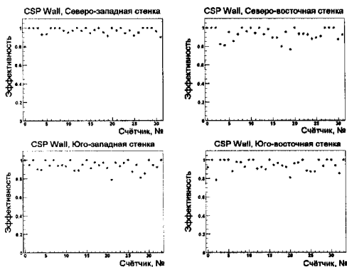
Рис. 6. Эффективности счётчиков CSP Wall.
