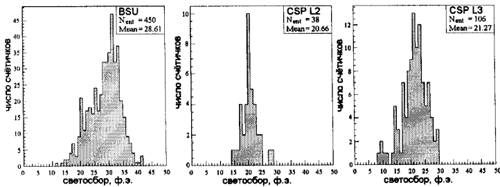
Рис. 9. Светосбор с дальнего от ФЭУ конца для синцилляционных счётчиков BSU, CSP L2 и CSP L3 типов, изготовленных в ОИЯИ.
