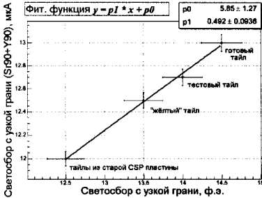
Рис. 15. Корреляция светосбора с узкой грани тайла, измеренного разными способами: методом абсолютной калибровки и с помощью радиоактивного источника, который был установлен в центре тайла.
