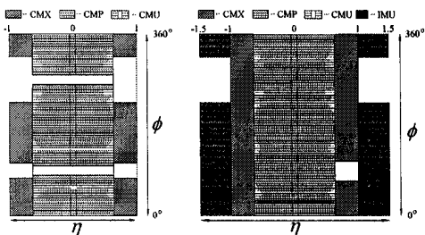
Рис. 11. Аксептанс мюонной системы CDF в Run I – слева и в Run II – справа.
