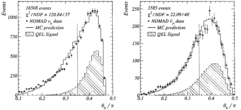
Рис. 5: Распределение \theta_h для 1-трековых \nu_\mu и \bar{\nu}_\mu событий.
