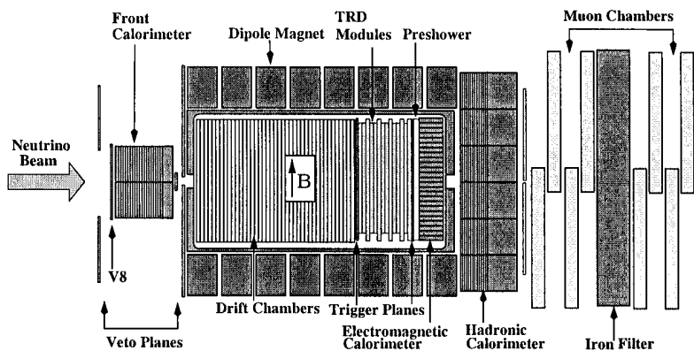
Рис. 1: Детектор NOMAD (вид сверху).
