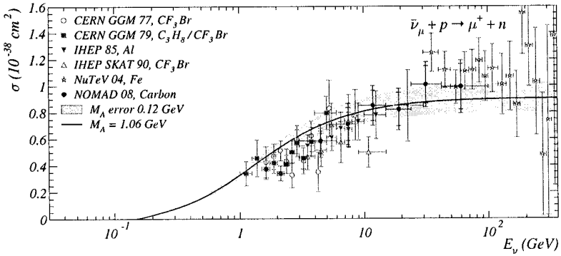
Рис. 8: Сравнение полученных результатов с данными предыдущих экспериментов. Сплошная линия соответствует значению аксиальной массы, полученному при анализе данных эксперимента NOMAD по \bar{\nu}_\mu рассеянию; заштрихованная область - полной ошибке; расчет выполнен для углерода согласно модели Smith-Moniz.
