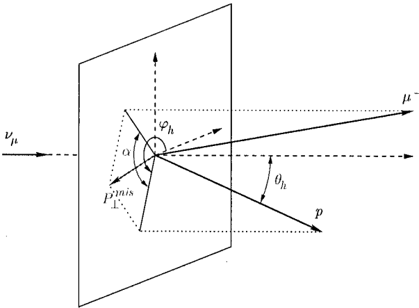
Рис. 3: Переменные, используемые в функции правдоподобия \mathcal{L} : недостающий поперечный импульс P_{\perp}^{mis} , угол вылета протона \theta_h , угол \alpha между поперечными компонентами импульсов заряженных треков. Также показан азимутальный угол протона \varphi_h .
