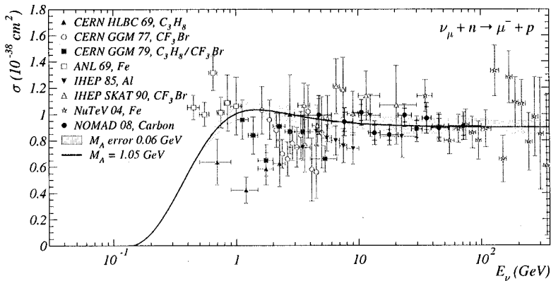
Рис. 6: Сравнение полученных результатов (приведена статистическая и полная ошибка измерения для каждого интервала E_\nu ) с данными предыдущих экспериментов на ядерной мишени. Сплошная линия соответствует значению аксиальной массы, полученному при анализе данных эксперимента NOMAD по \nu_\mu рассеянию; заштрихованная область - полной ошибке. Расчет выполнен для углерода согласно модели Smith-Moniz.
