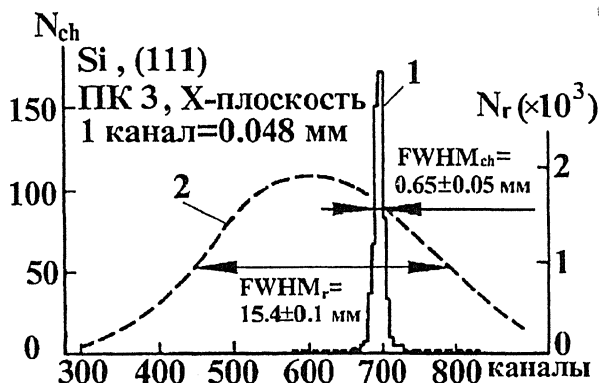
Рис.12. Пространственное расположение пучка на X плоскости (ПКЗ): 1 — с отбором по критерию малой амплитуды сигнала с детектора (в интервале 0.3 \div 0.6 от наиболее вероятного значения для хаотической фазы), 2 — без отбора (прямой пучок).
