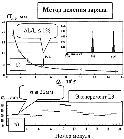
Рис.15. Пространственное разрешение ФТС.
