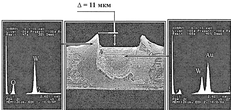
Рис.21. Типичные результаты обследования анодной проволоки методом SEM/XEM в точке, расположенной вблизи зоны облучения со стороны выхода газового потока. Очень толстый слой ( 11мкм ) окиси вольфрама хорошо наблюдается поверх золотого покрытия проволоки. Диаметр проволоочки – 30мкм.
