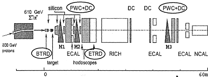
Рис.10. Блок-схема экспериментальной установки. BTRD – пучковый детектор переходного излучения (ДПИ); ETRD – электронный детектор переходного излучения (ДПИ); EMCL – электромагнитный калориметр; PWC – пропорциональные камеры; DC – дрейфовые камеры; RICH – черенковский детектор; NCAL – нейтронный калориметр; M1, M2 и M3 –анализирующие магниты.
