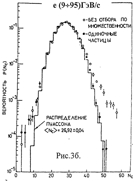
Рис.3. Распределение по числу зарегистрированных кластеров для \pi^- - мезонов (Рис.3а) и для электронов (Рис.3б).
