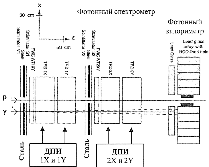
Рис.7. Фотонный спектрометр. Положение электромагнитного ливня в стальном конверторе измеряется пропорциональными камерами (PWC) и ДПИ (TRD). Энергия фотонов измеряется в фотонном калориметре.
