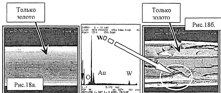
Рис.18. Эффект распухания анодной проволоочки. Рис.18а. Край проволоочки. Необлученная зона, X = -14 см. Диаметр – 35 мкм.
