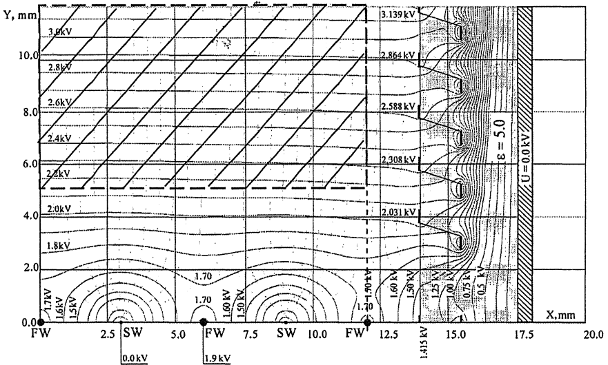
Рис.14. Компьютерная симуляция структуры электрического поля в модуле ФТС при наличии двух слоёв полеформирующих стрипови заземлённого защитного экрана, установленного в 3,5 мм от границы внутреннего объёма. Внешний слой стрипов смещён на 1 мм вниз относительно внутреннего.
