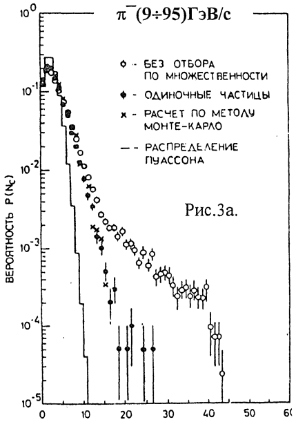
Рис.3. Распределение по числу зарегистрированных кластеров для \pi^- - мезонов (Рис.3а) и для электронов (Рис.3б).
