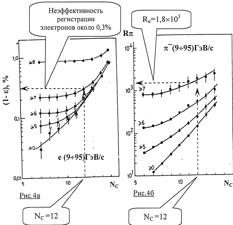
Рис.4. Неэффективность регистрации электронов (Рис.4а) и величина коэффициента режекции \pi^- -мезонов (Рис.4б) как функция от порога по числу зарегистрированных кластеров для разных значений порога по числу сработавших камер ДПИ.
