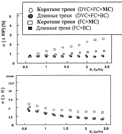
Рис. 17. Импульсное и угловое разрешения, полученные для коротких и длинных треков, при различных комбинациях использования информации с различных трековых детекторов.
