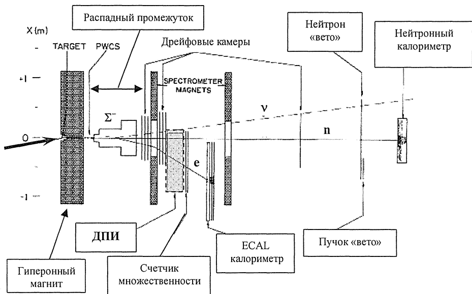
Рис.1. Экспериментальная установка по исследованию \beta распада \Sigma^- гиперонов.
