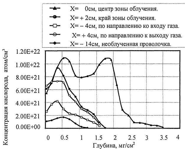
Рис.19. Распределение концентрации кислорода как функция глубины золотого покрытия в различных точках вдоль анодной проволоки. Ориентировочный масштаб: 1мг/см 2 соответствует 0,5мкм по толщине.
