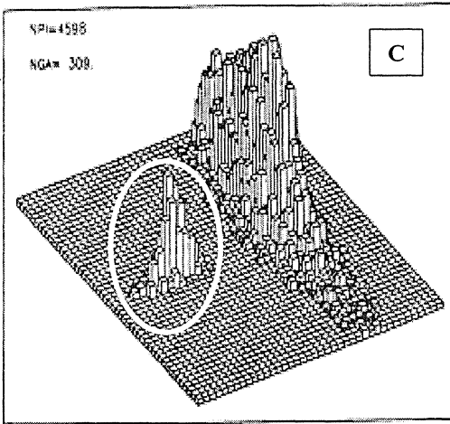
Рис.9. Распределение \chi^2 ДПИ как функция от величины M_{\chi^0}^2 в виде трехмерного распределения полученных событий.
