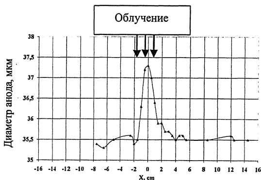
Рис.20а. Эффект распухания анодной проволочки. Зависимость диаметра проволочки от координаты вдоль проволочки.
