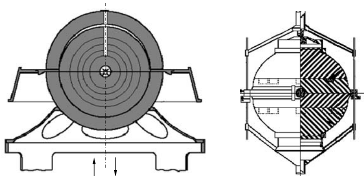
Рис. 5. Вид в разрезе плутониевыхборок «Jezebel» (слева) и ВНИИЭФ (справа)
