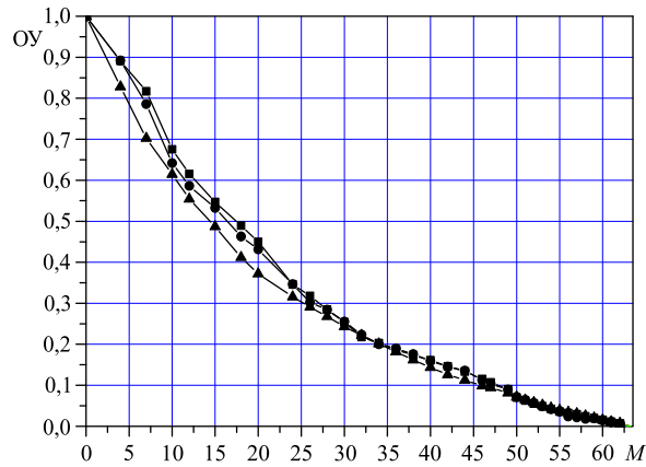
Рис. 3. Экспериментальная зависимость ОУ от числа загруженных в АЗ ТВС ( M ) для трех пусковых каналов ( \blacktriangle , \bullet , \blacksquare ). Экстраполированное число ТВС равно 63
