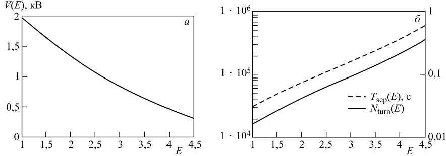
Рис. 2. Зависимость параметров сепаратрисы от энергии ионов (ГэВ/нукл.): а) амплитуда барьерного ВЧ-напряжения V(E) (1.10); б) число оборотов (сплошная кривая) и период обращения (штриховая кривая, с) ионов золота ^{197}\text{Au}^{79+} при движении по сепаратрисе; параметры накопителя и ВЧ-системы: периметр C_{\text{Ring}} = 503 м, \gamma_{\text{tr}} = 7,09 , |\Delta p/p_s| = 5 \cdot 10^{-4} , \Delta\varphi_B = \pi/10 , \Delta\varphi_{BB} = 1,3\pi^*
