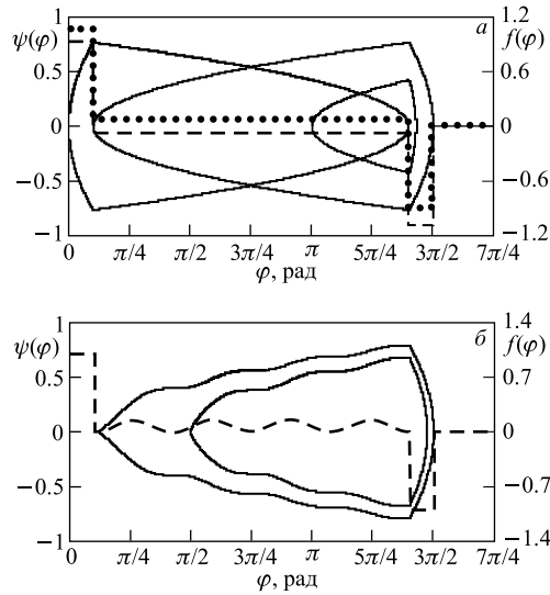
Рис. 13. Влияние разностей значений V_{\text{acc}}(\varphi) и |V_{\text{dec}}(\varphi)| на фазовое движение частиц при ускорении: а) \delta f_B(\varphi) = \text{const} во всей фазовой области (3.4), точечная кривая — \delta f_B(\varphi) > 0 , штриховая кривая — \delta f_B(\varphi) < 0 , две правые сплошные кривые — сепаратриса и промежуточная фазовая траектория при \delta f_B(\varphi) > 0 , левая сплошная кривая — сепаратриса при \delta f_B(\varphi) < 0 ; б) штриховая кривая — \delta f_B(\varphi) = f_d \left( 1 - \cos 8\pi \frac{\varphi - \Delta\varphi_B}{\Delta\varphi_{BB}} \right) , f_d = \Delta\varphi_B / \Delta\varphi_{BB} , сплошные кривые — сепаратриса и промежуточная фазовая траектория; условие (4.10) выполняется во всех случаях
