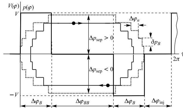
Рис. 1. Схема движения частицы в фазовом пространстве p(\varphi) между импульсами барьерного напряжения прямоугольной формы (жирная сплошная кривая); тонкая сплошная кривая — стабильная фазовая траектория p(\varphi) ; точечная кривая — сепаратриса; функции p(\varphi) и V(\varphi) даны в произвольных единицах; \varphi_s = 2\Delta\varphi_B + \Delta\varphi_{BB}
