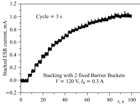
Рис. 8. Накопление ионов ^{124}\text{Xe}^{54+} в ESR [10] с барьерной ВЧ-системой и электронным охлаждением. Насыщение интенсивности накопленных частиц связано, видимо, с несовершенством применяемой ВЧ (подразд. 3.5)
