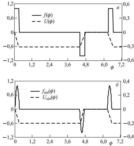
Рис. 3. Функции f(\varphi) (сплошные кривые) и U(\varphi) (штриховые кривые) для прямоугольных (а) и квазисинусоидальных (б) барьеров; \Delta\varphi_B = \pi/10 , \Delta\varphi_{BB} = 1,3\pi
