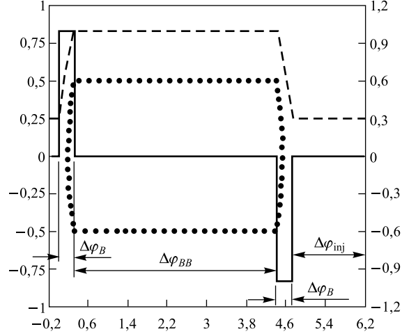
Рис. 6. Фазовые траектории инжектированной частицы (штриховая кривая, \varphi_{inj} = -0,2 , Y_{inj} = 0,25 ) и частицы, захваченной в потенциальную яму области накопления (точечная кривая, Y_{max} = 0,5 ), f(\varphi) — сплошная кривая
