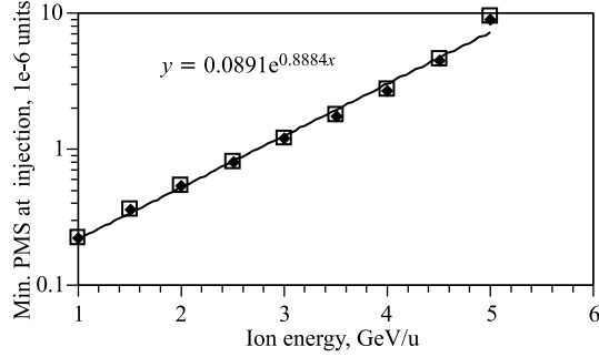
Рис. 7. Зависимость |\Delta p_{inj}|/p_s (в единицах 10^{-6} ) от энергии частицы; ромбиками показаны результаты численного решения уравнения (3.10), (3.11) для случая прямоугольных барьеров, а светлые квадраты — приближенные значения по формуле (3.12); параметры накопителя и барьерной системы те же, что и в предыдущих примерах, |\Delta p/p_s|_{sep} = 5 \cdot 10^{-4} , T_{inj} = 10 с; формула аппроксимации показана на рисунке
