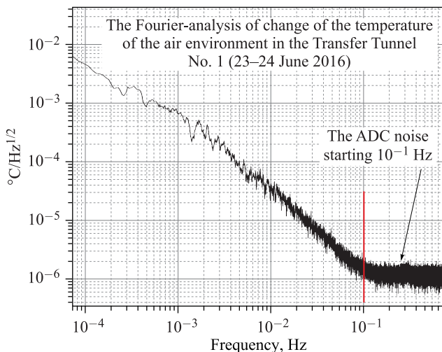
Рис. 6. Фурье-анализ изменений температуры воздуха в транспортном тоннеле № 1 по данным рис. 4
