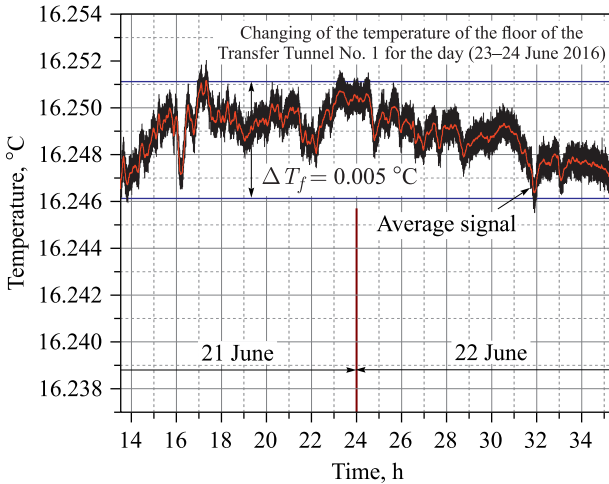
Рис. 5. Суточное изменение температуры бетонного пола в транспортном тоннеле № 1 с 21 по 22 июня 2016 г.
