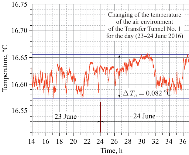
Рис. 4. Суточное изменение температуры воздуха в транспортном тоннеле № 1 с 23 по 24 июня 2016 г.
