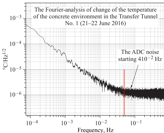
Рис. 7. Фурье-анализ изменений температуры бетонного пола транспортного тоннеля № 1 по данным рис. 5
