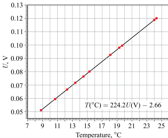
Рис. 3. Зависимость сигнала с термистора от внешней температуры
