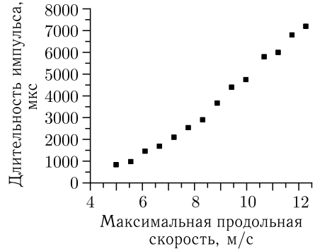
Рис. 7. Ширина импульса, формируемого линзой, в зависимости от максимальной продольной скорости
