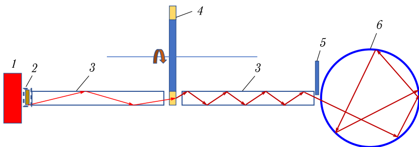
Рис. 3. Принципиальная схема источника: 1 — основной замедлитель; 2 — замедлитель-конвертер; 3 — нейтронотвод; 4 — временная линза с дифракционными решетками; 5 — быстрый клапан; 6 — ловушка-накопитель
